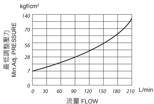
最低調整壓力-最大流量特性 Min.Adj. PRESSURE v.s. MAX. FLOW
