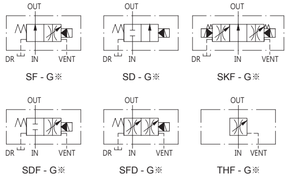
閥類型符號 SYMBOL
